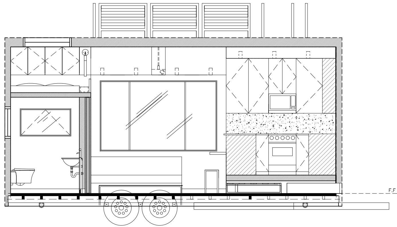
1 SECTION 3 SCALE: 1/4" = 1'-0"
