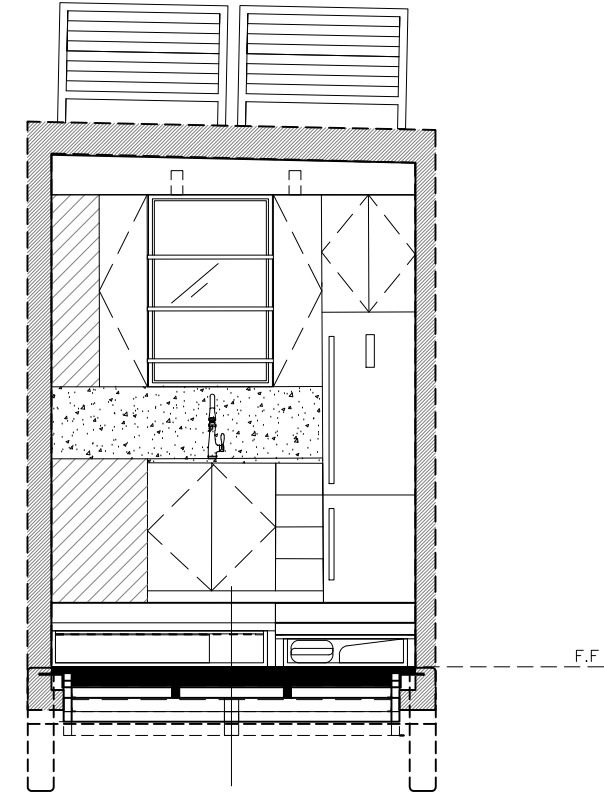
2 SECTION 2 SCALE: 1/4" = 1'-0"
