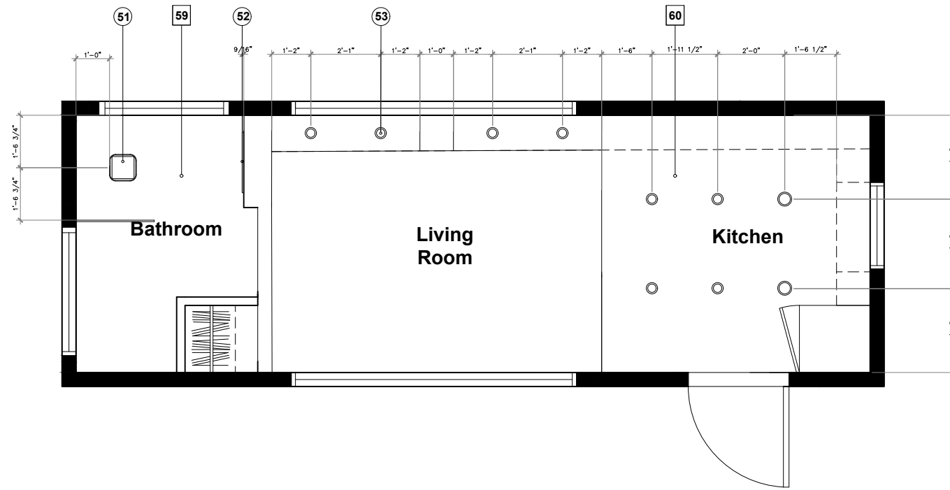
② RCP LEVEL 1 SCALE: 1/4" = 1'-0"
