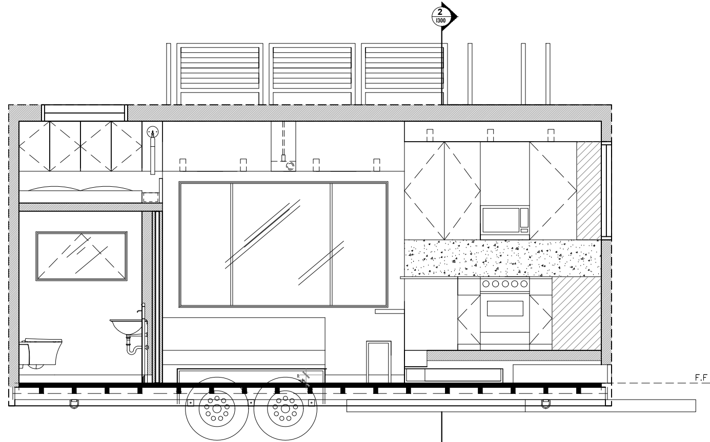
3 SECTION 1 SCALE: 1/4" = 1'-0"
